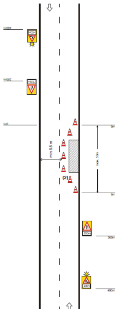
Εικόνα 7. Στένωση λωρίδας σε αστική οδό με μικρή κυκλοφορία
