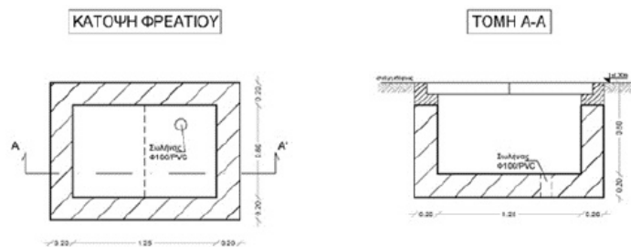
Εικόνα 2. Φρεάτιο διαστάσεων 1,25X0,80X0,80
