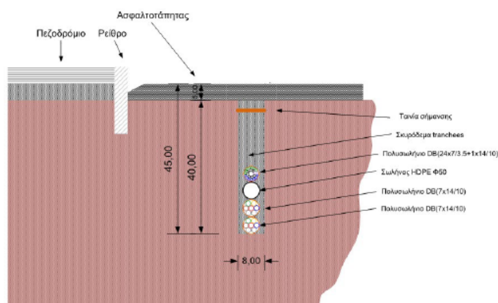
Εικόνα 1. Τομή τάφρου 0,08μ. x 0,45μ. επί οδοστρώματος.
