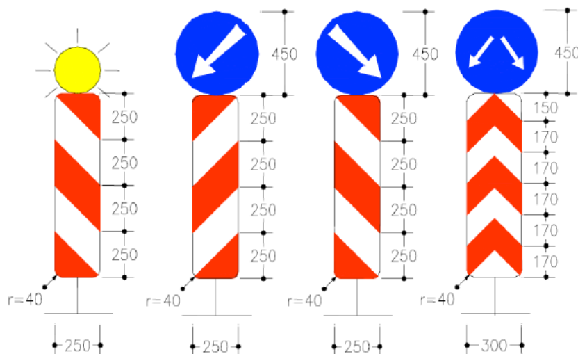
Εικόνα 5. Διαστάσεις πινακίδων οριοθέτησης διαδρόμου κυκλοφορίας
