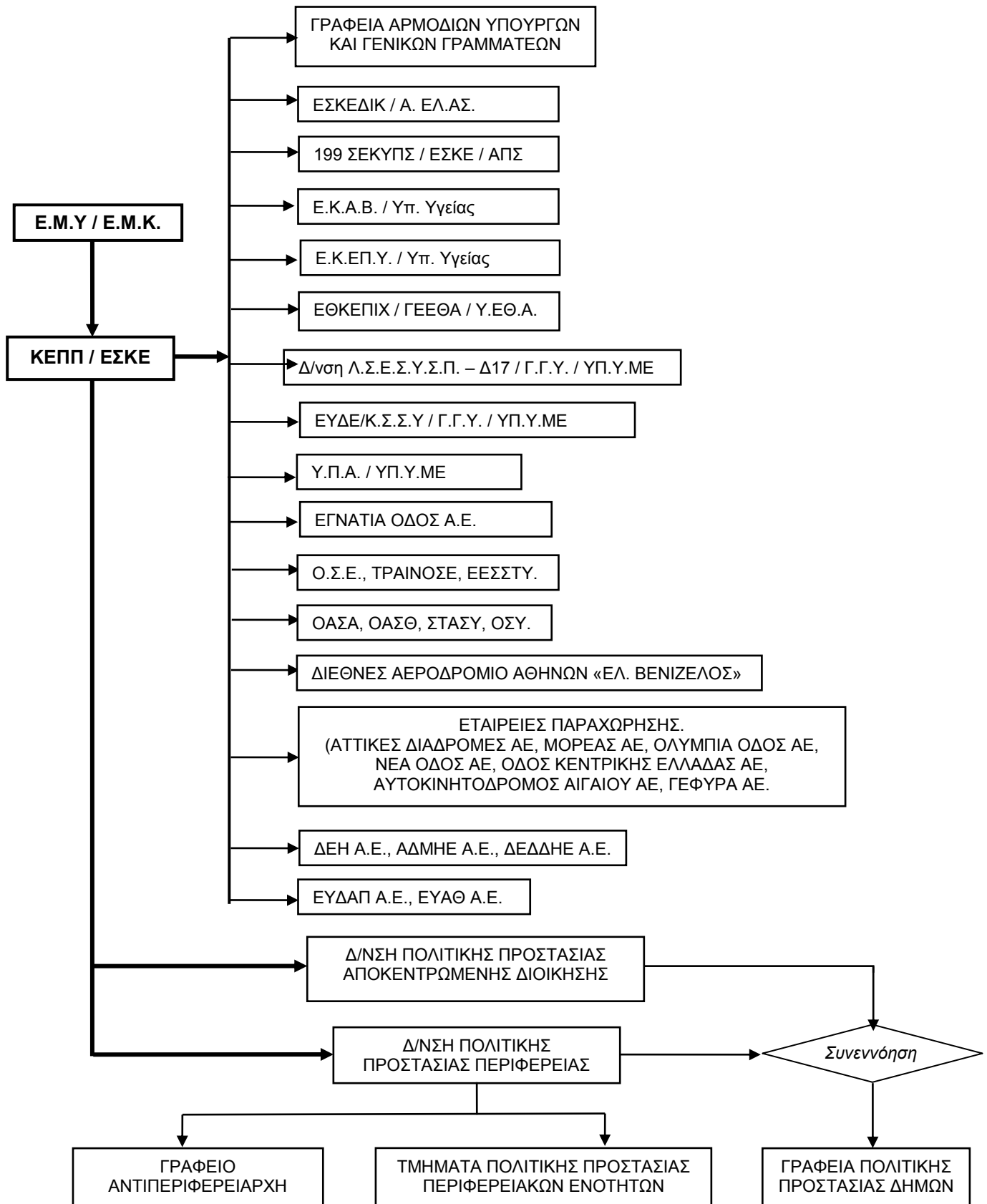
Διάγραμμα 1. Διάγραμμα ροής αποστολής των Έκτακτων Δελτίων της ΕΜΥ 17 και ιδιαίτερου προειδοποιητικού σήματος από το ΚΕΠΠ/ ΕΣΚΕ
